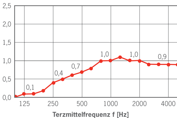
Äquivalente Schallabsorptionsfläche [m 2 ] Holzrahmen mit bedrucktem Stoff (1200 x 800 x 30 mm)
