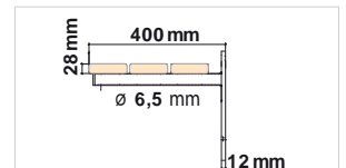
6210 - Bankkonsole mit Wandbefestigung
