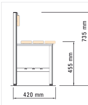
R 6250 - Bankkonsole mit Gleitfüßen oder Bodenbefestigung, integrierter Rückenlehne, Schuhrost optional
