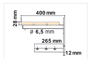
6220 - Bankkonsole mit Wandbefestigung und Schuhrost
