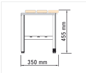
R 6240 - Bankkonsole mit Gleitfüßen oder Bodenbefestigung, Schuhrost optional
