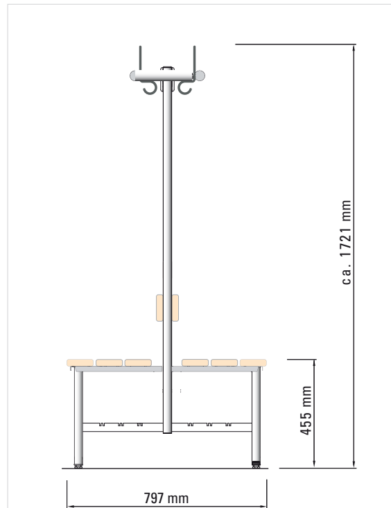
R 6680 - beidseitige Umkleidebank mit Garderobe 1600, mit zwei Rückenlehnen, Schuhrost optional. Haken frei wählbar (mit 1800 Wandgarderobe R 6880)
