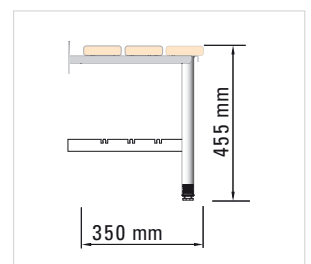
R 6230 - Bankkonsole mit Wand und Bodenbefestigung, Schuhrost optional
