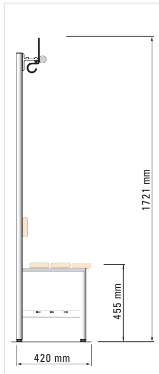
R 6670 - einseitige Umkleidebank mit Garderobe 1600, mit Rückenlehne, Schuhrost optional. Haken frei wählbar (mit 1800 Wandgarderobe R 6870)
